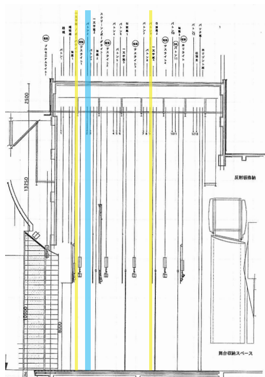
大ホール立面図
