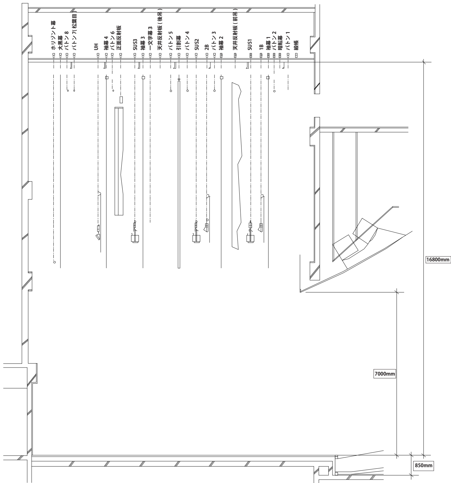
岩見沢市文化センター断面図 1/100 (A-4)
